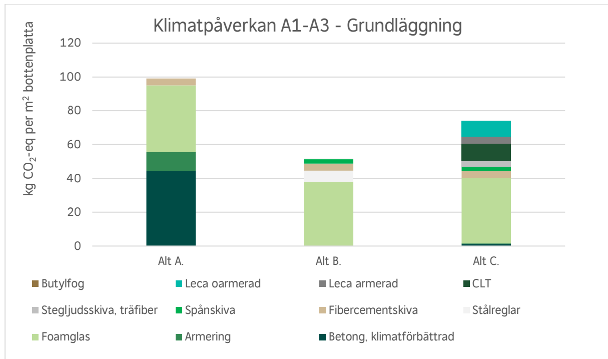
Figur 5. Resultat av jämförelsen avseende klimatpåverkan för de föreslagna alternativen för grundläggning.
